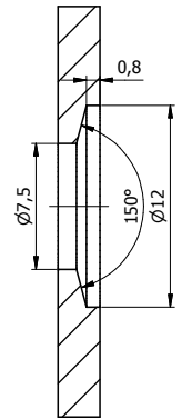
A-A (2 : 1)
